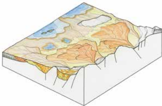
Reconstrucción paleoambiental de la provincia de Segovia durante el Mioceno, con los abanicos aluviales que desde la sierra arrastraban sedimentos hasta los lagos distales, en los que se formaron las calizas y margas de los páramos.
